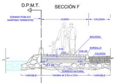
PLANO DE SECCIÓN DE LA ACERA MARÍTIMA
